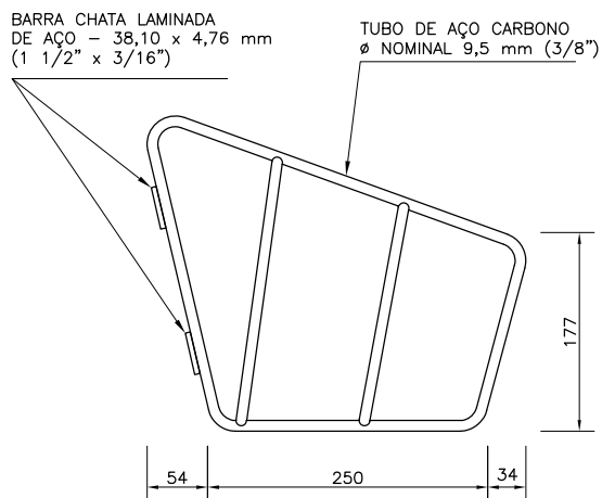
VISTA LATERAL
